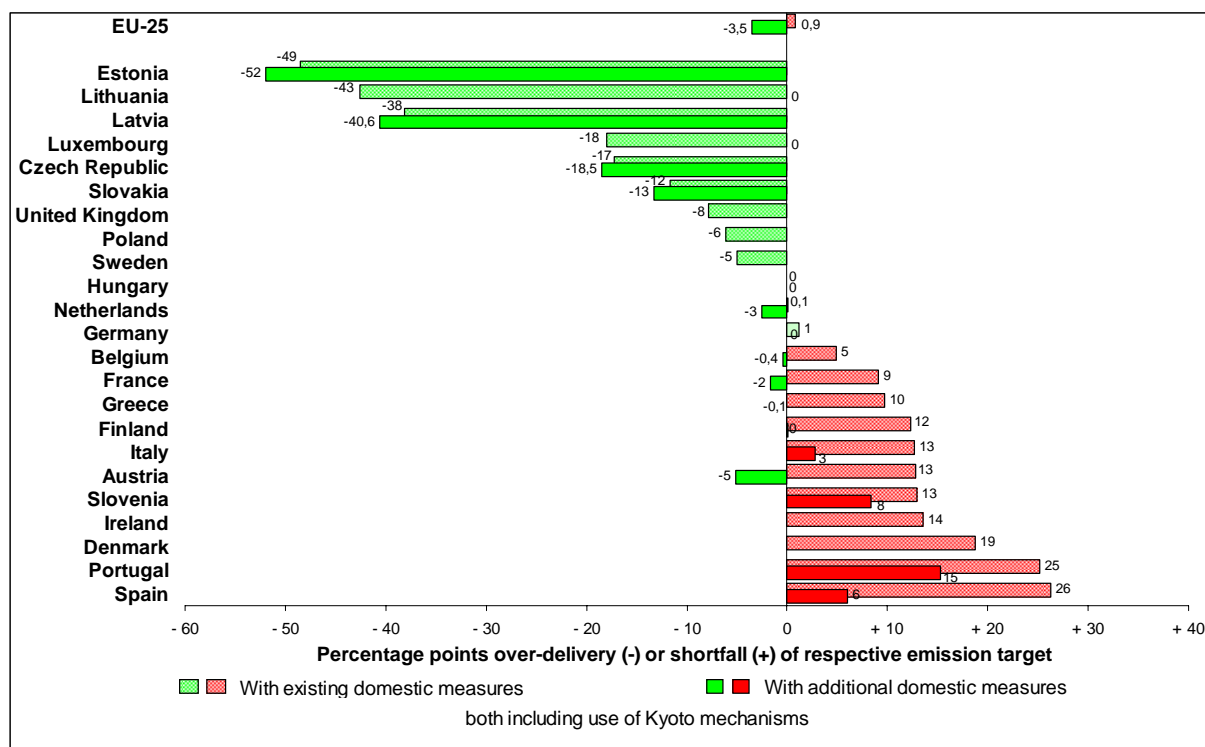
Figura 3: Id-distakk mill-miri fl-2010 (f'punti perċentwali) għall-UE-25, bil-mekkanizmi ta' Kyoto inkluzi
