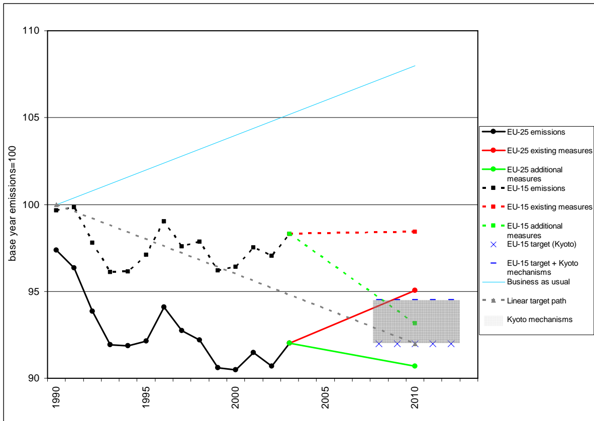
Figura 1: L-emissjonijiet attwali u projettati għall-UE-25 u l-UE-15
