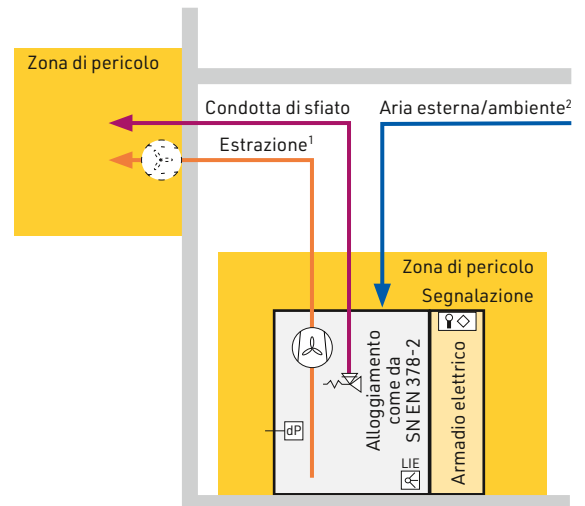
[FIG. 5] Schema esemplificativo di alloggiamento ventilato. Immagine: Scheco AG
