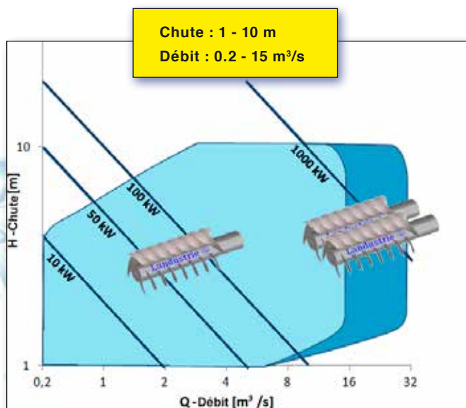
Plage de fonctionnement des turbines
