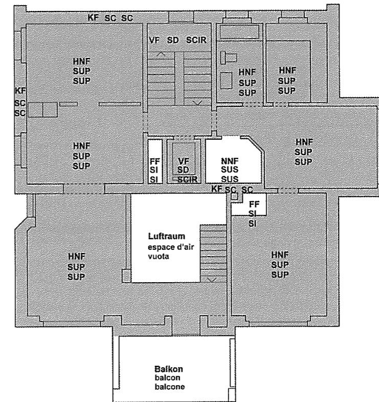
Figur 6 Anrechenbare Geschossflächen
