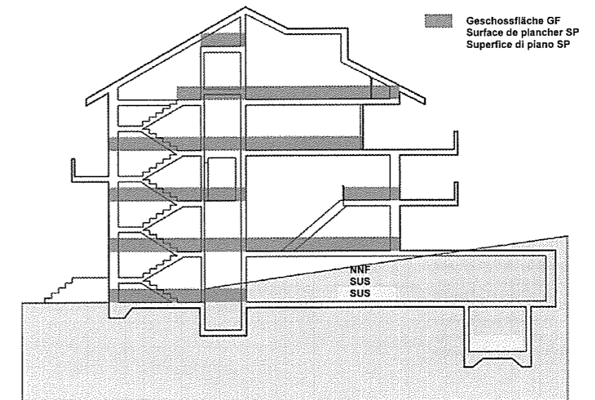
Figur 7 Anrechenbare Geschossflächen
