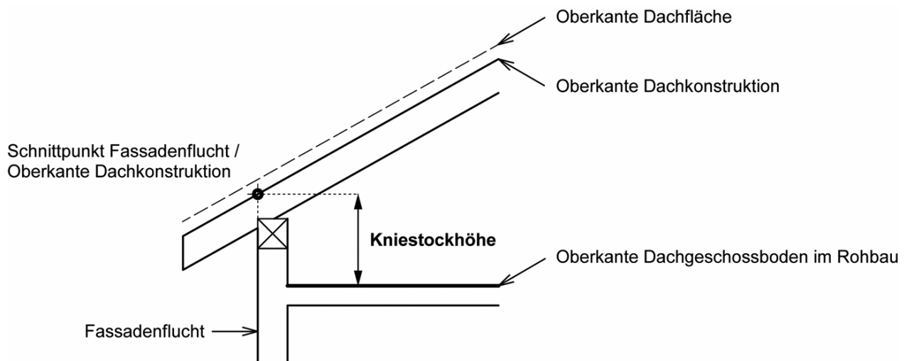
Figur 5.3 Kniestockhöhe
