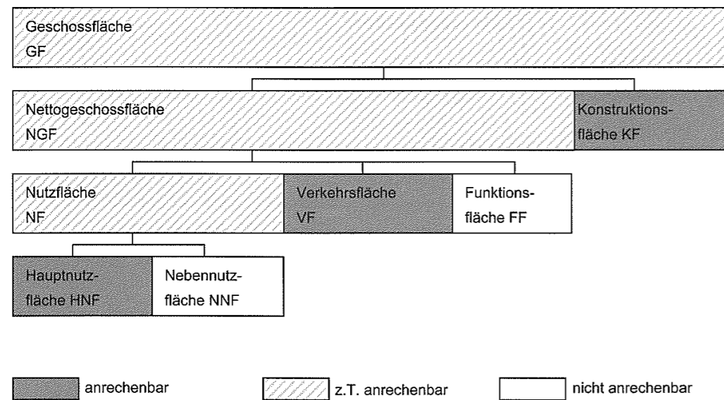
Figur 5 Anrechenbare Geschossflächen
