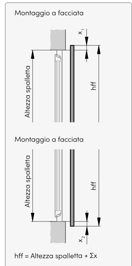
Altezza anta (hff), persiana scorrevole/persiana scorrevole Vento
