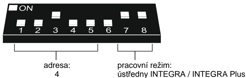
Obr. 7. Příklad nastavení DIP-přepínačů.
